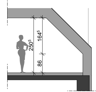
SCHNITT 2-2
