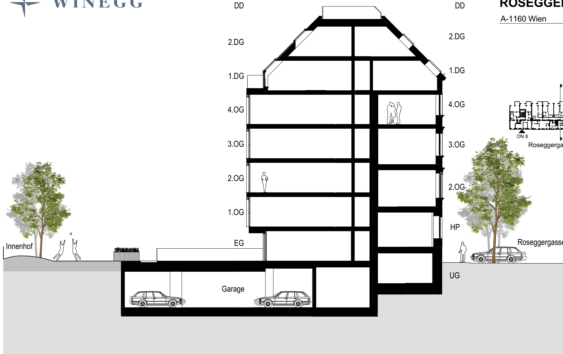
Schnitt Roseggergasse
