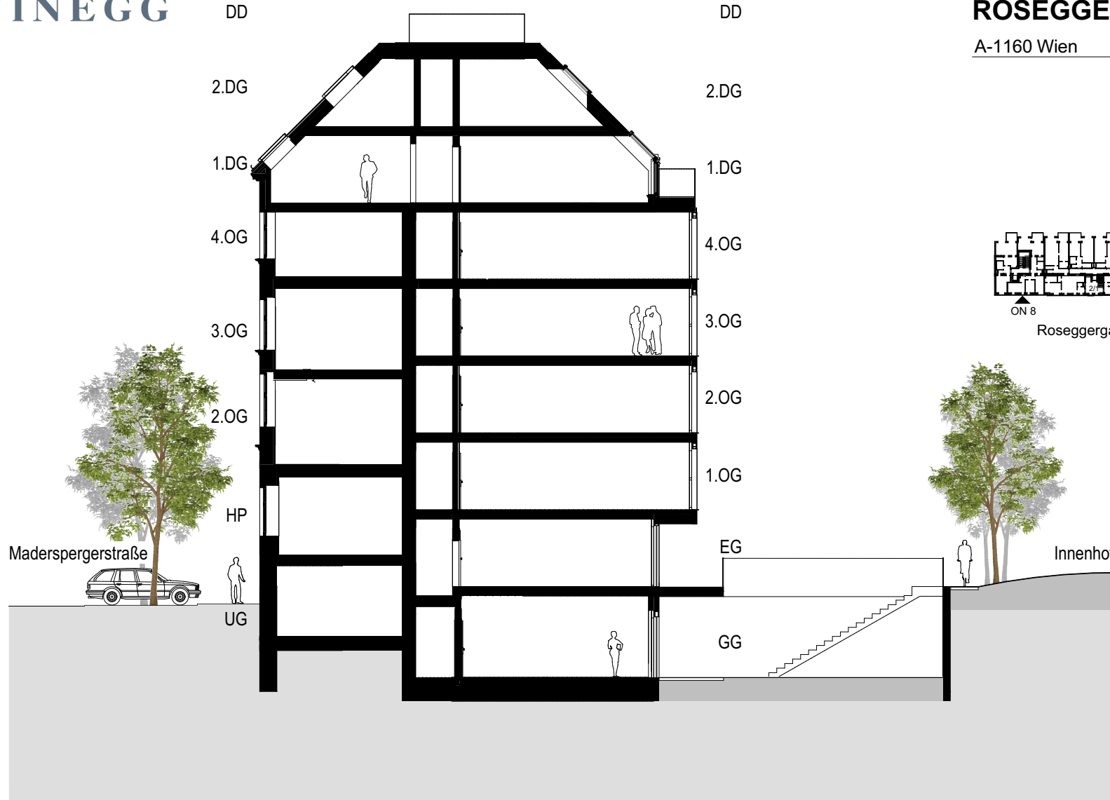
Schnitt Maderspergerstraße
